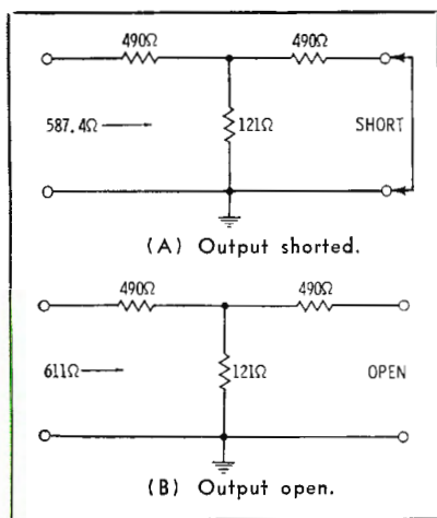
Fig. 5. A twenty-decibel loss network.
