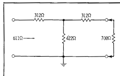
Fig. 3. Ten-decibel T pad, 700-ohm load.
